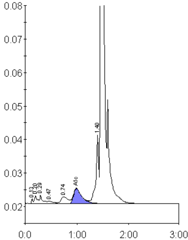
Peak table - ID: 10563887
